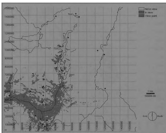
Ryc. 11. Wynik „analizy widoczności” – (fragment) rzeka Główna (3 m/6600 m)
