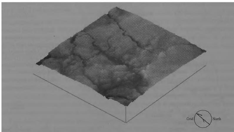
Ryc. 3. Cyfrowy Model Terenu obszaru Ostrowa Lednickiego
