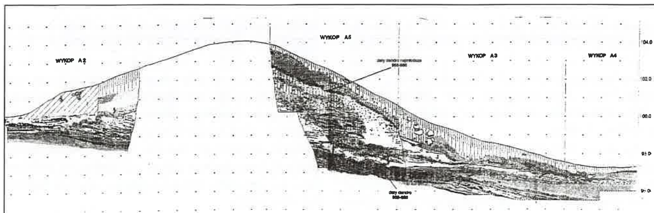
Ryc. 13. Giecz – badania archeologiczne wału, przekrój ok. 2000 (rys. T. Krysztofiak) Fig. 13. Giecz – archaeological research of the rampart, cross-section ca. 2000 (drawing by T. Krysztofiak)
